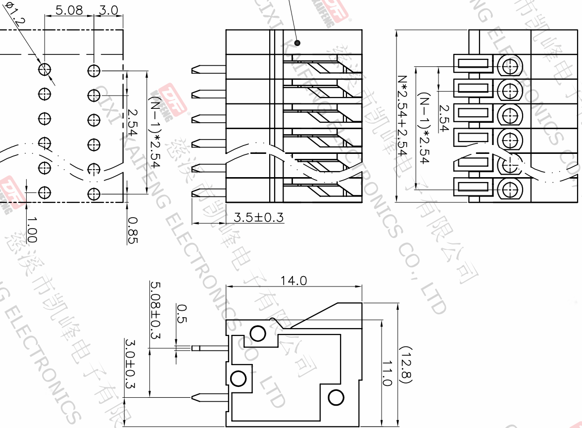
P.C.B.LAYOUT
