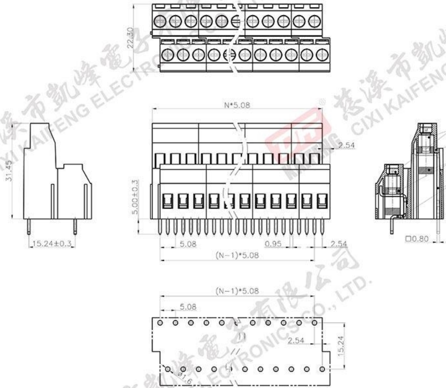
P.C.B LAYOUT
