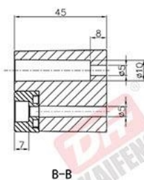
防呆结构
